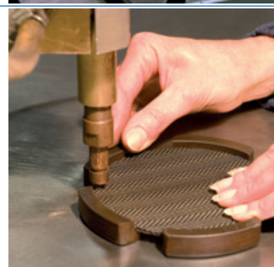
Punktschweißen
